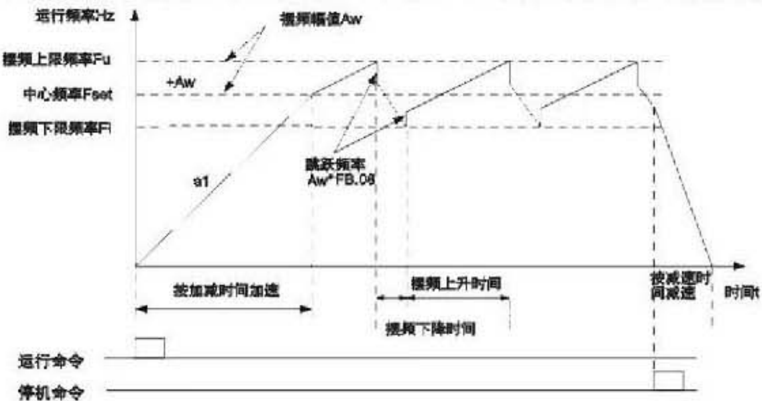
图FB-1 摆频示意图
