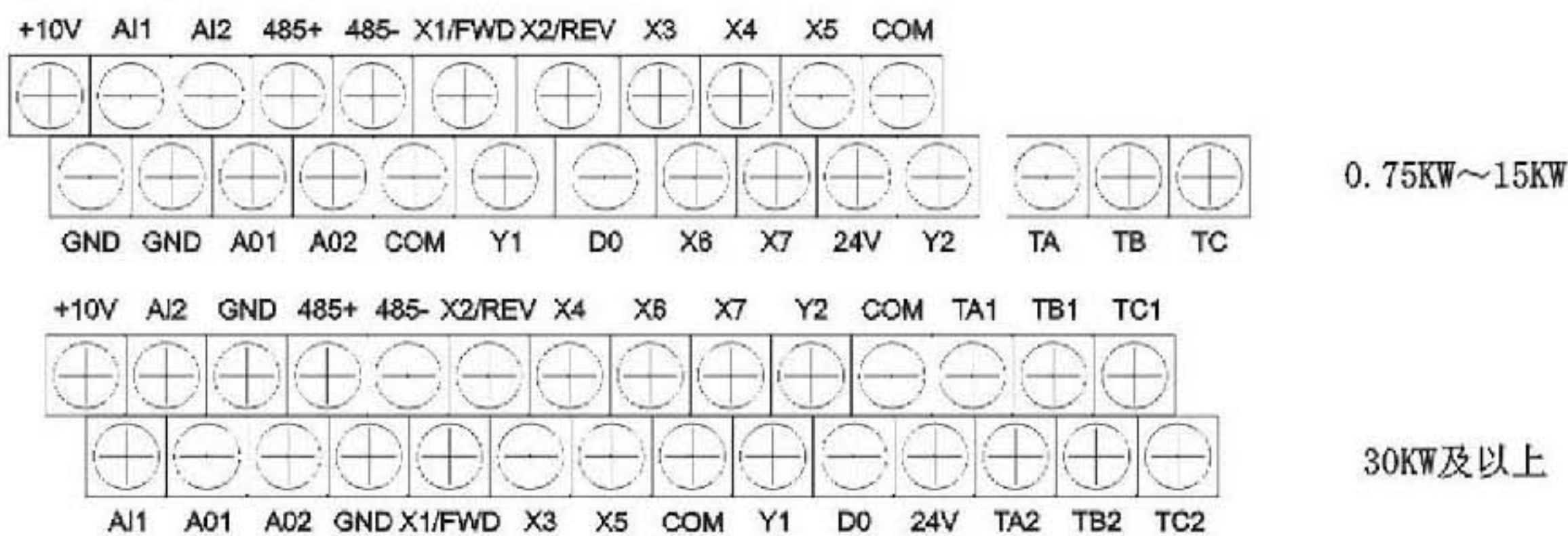
控制回路端子功能说明
