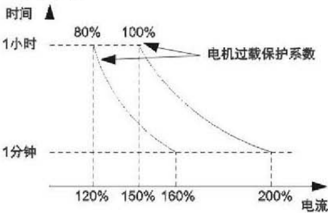
图F9-2 电机过载保护系数设定示意图
