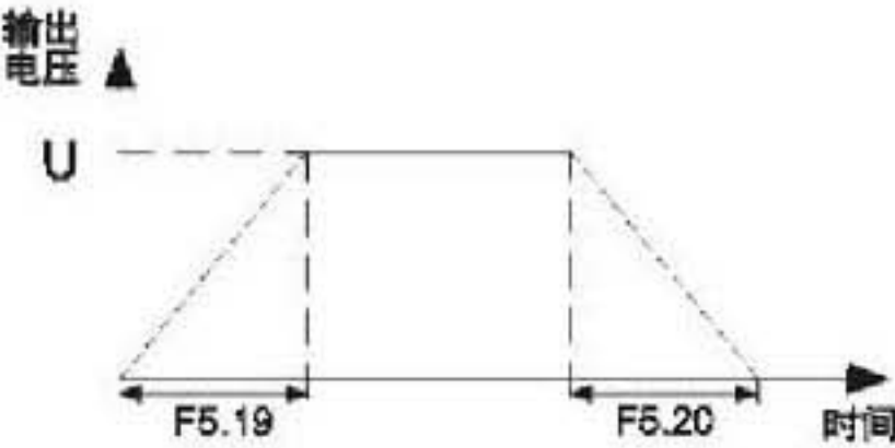
图F3-6 电压控制模式1
