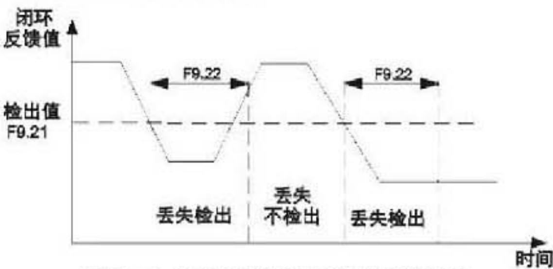
图F9-4 闭环反馈丢失检出时序图
