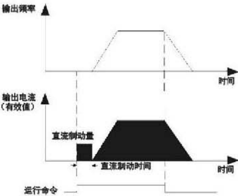
图F6-2 起动直流制动示意图
