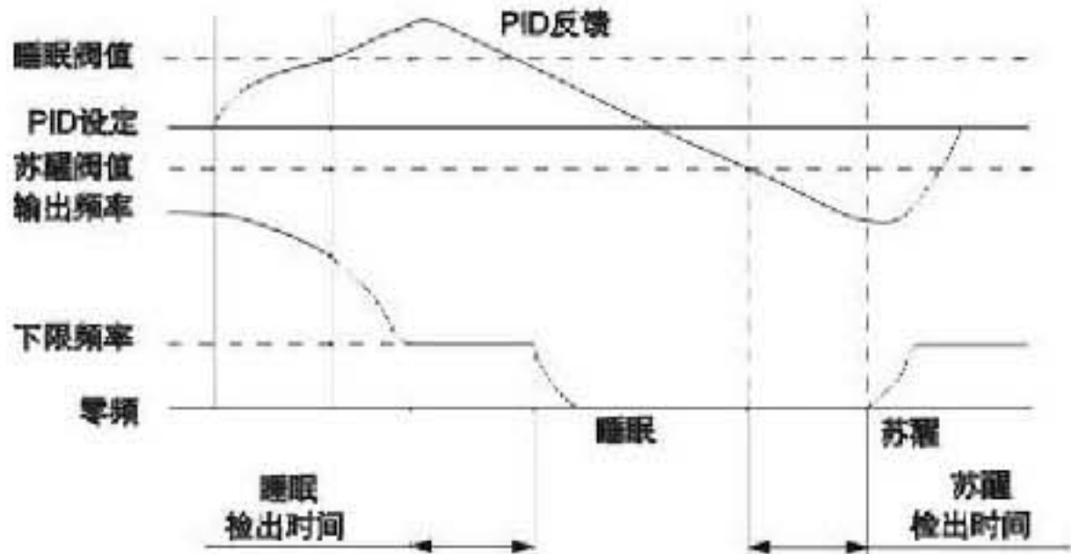
图FA-5 第一种睡眠模式示意图
