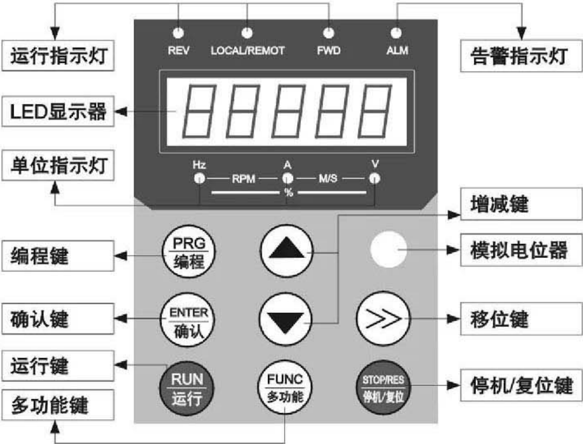
键盘示意图
