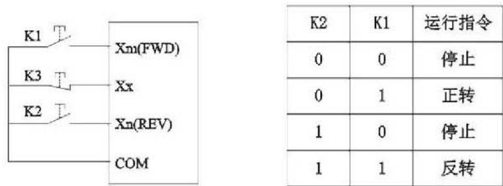
图F4-5 三线式控制模式2示意图
