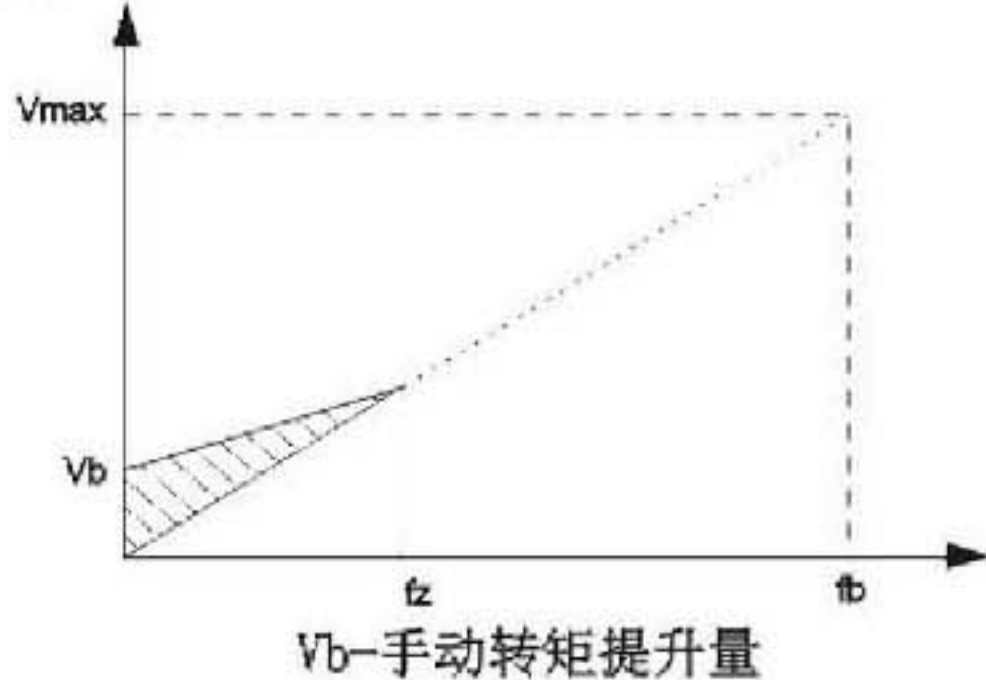
图F3-3 转矩提升示意图
