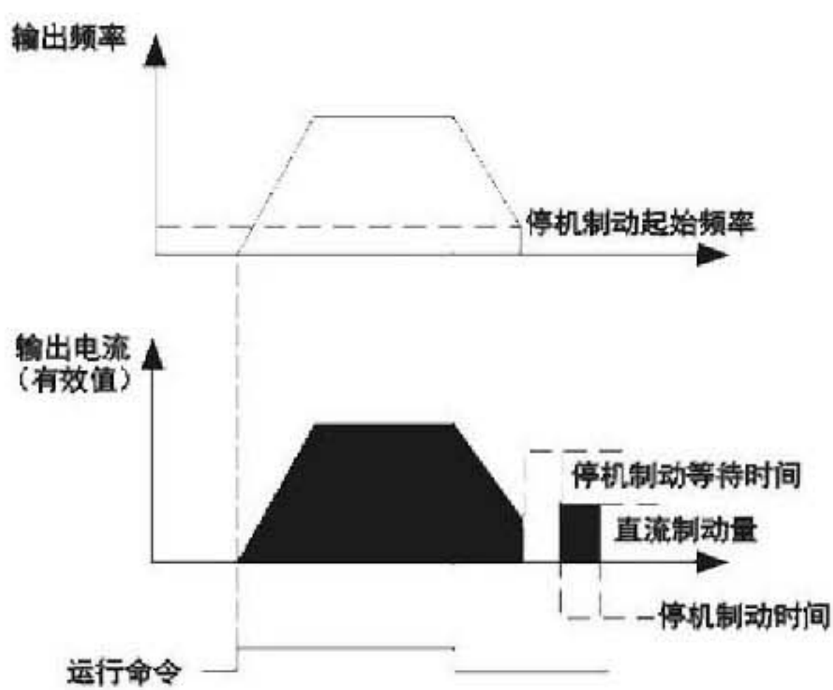
图F6-4 停机直流制动示意图
