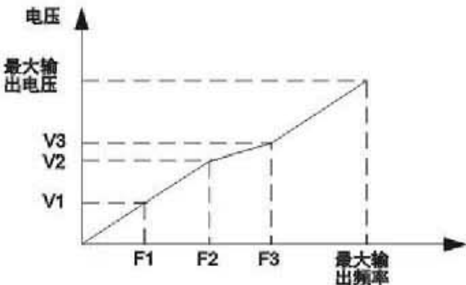
图F3-4 用户设定V/F曲线示意图
