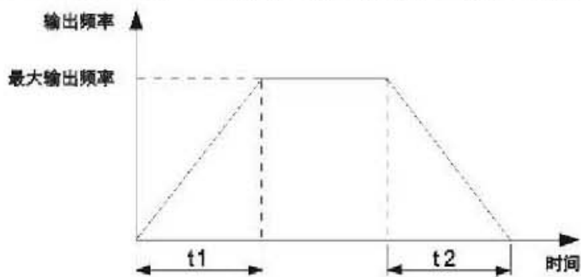
图F0-2 加速时间和减速时间示意图
