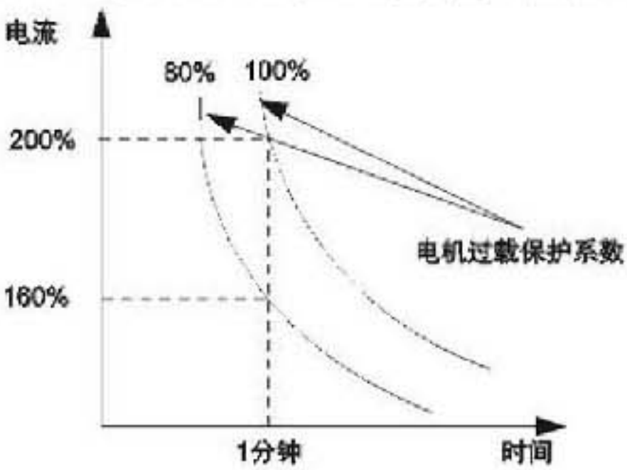
图F9-1 电机过载保护曲线
