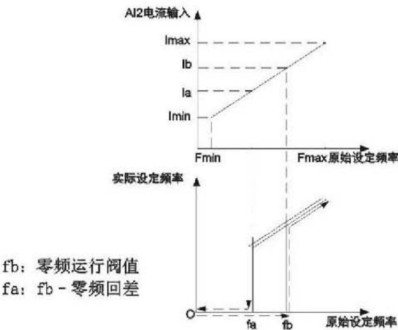
图F4-6 零频功能示意图
