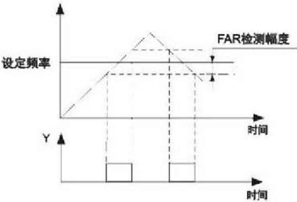
图F8-4 频率到达示意图
