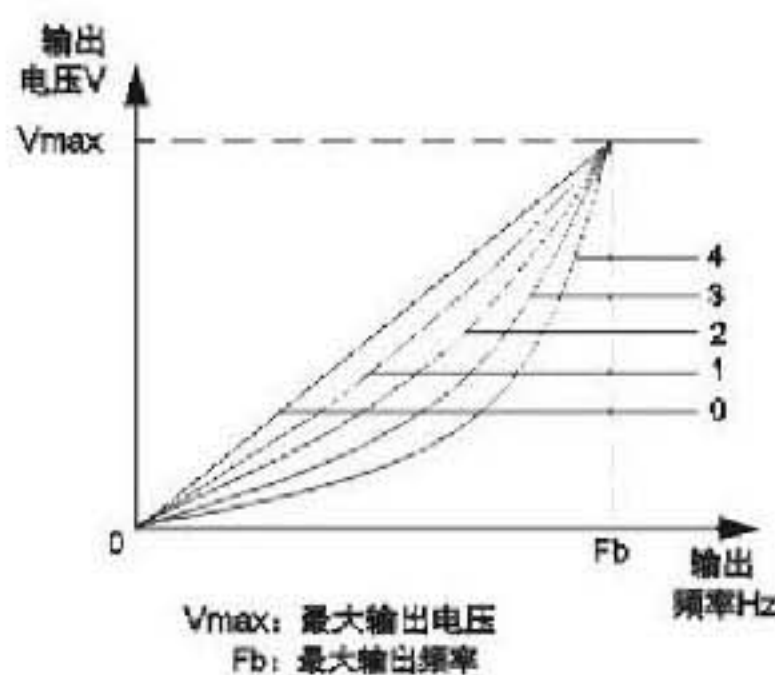
图F3-1 V/F曲线示意图
