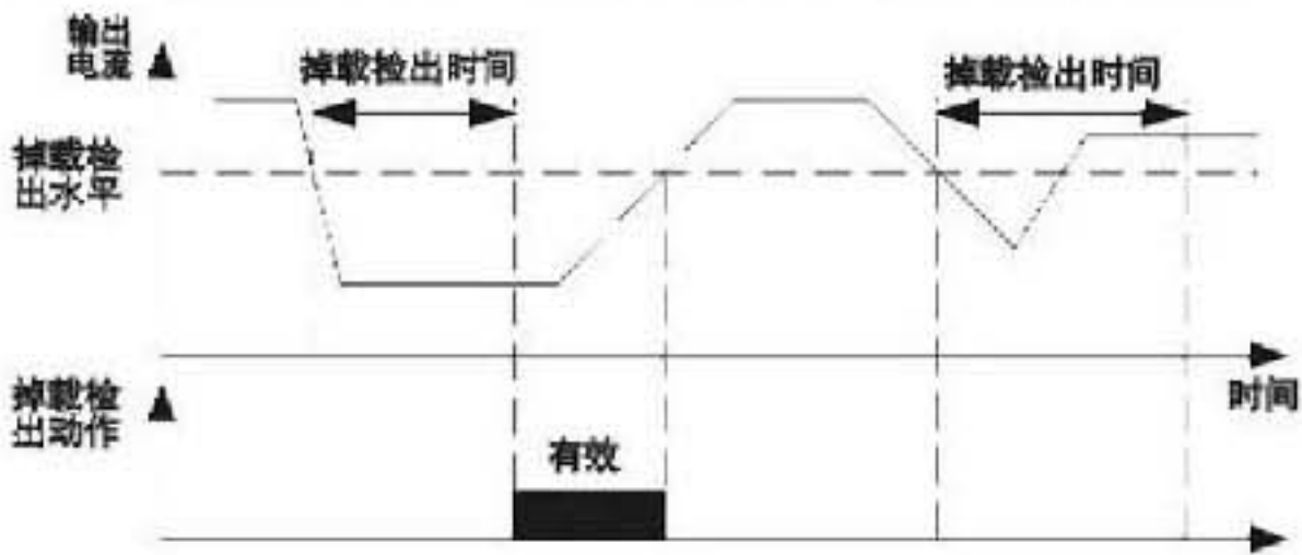
图F9-3 掉载检出示意图
