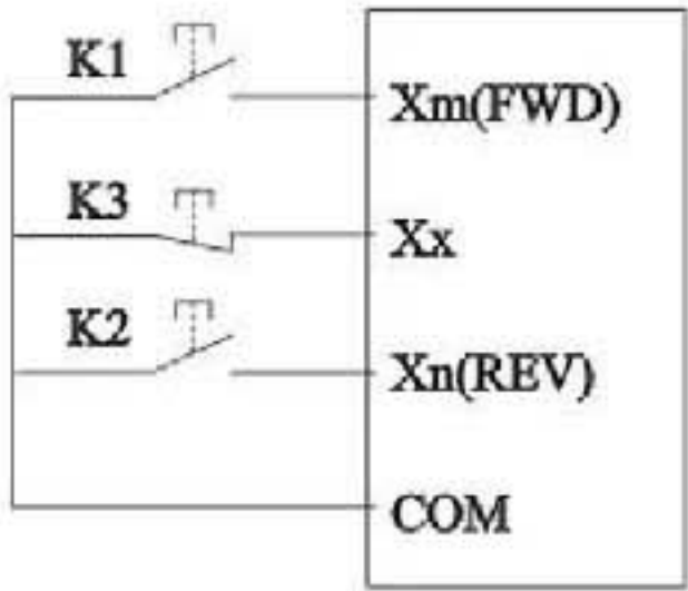
图F4-4 三线式控制模式1示意图
