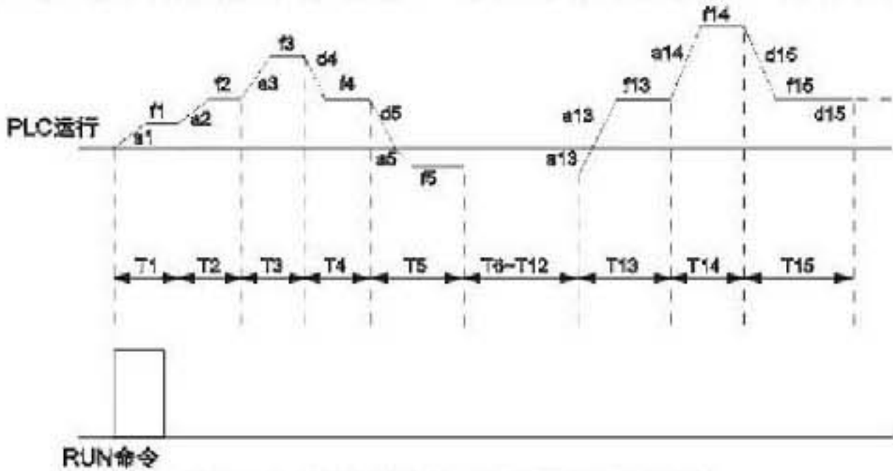
图FC-2 PLC单循环后保持示意图
