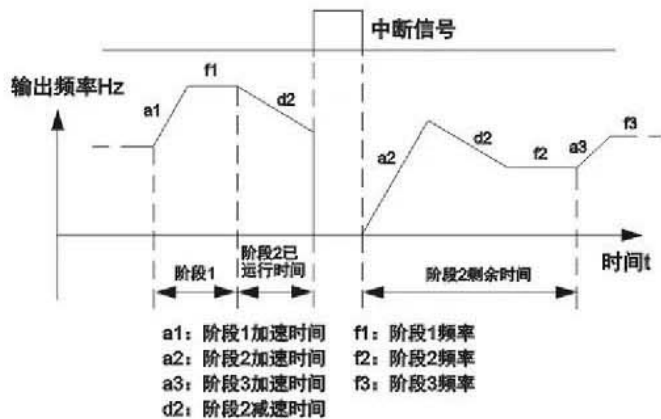
图FC-5 PLC启动方式2
