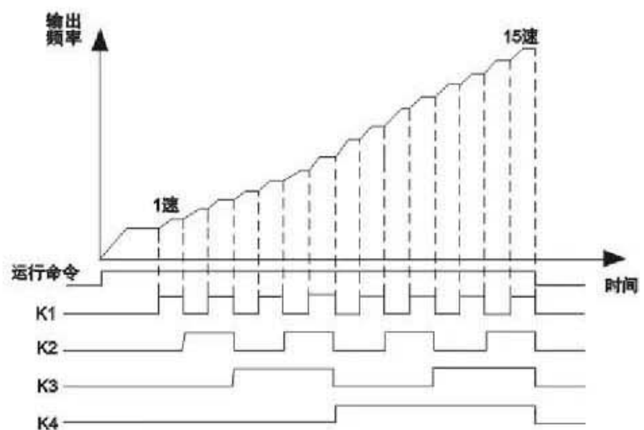
图F4-1 多段速运行示意图
