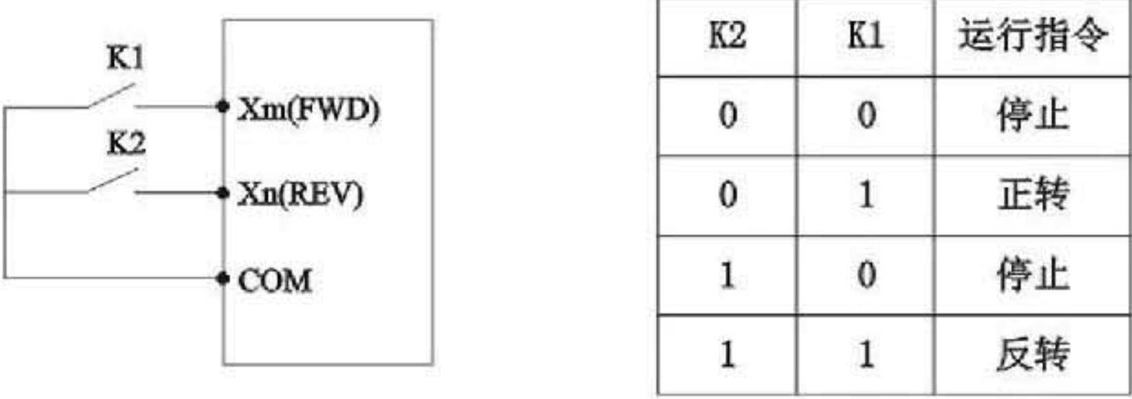
图F4-3 二线式控制模式2示意图
