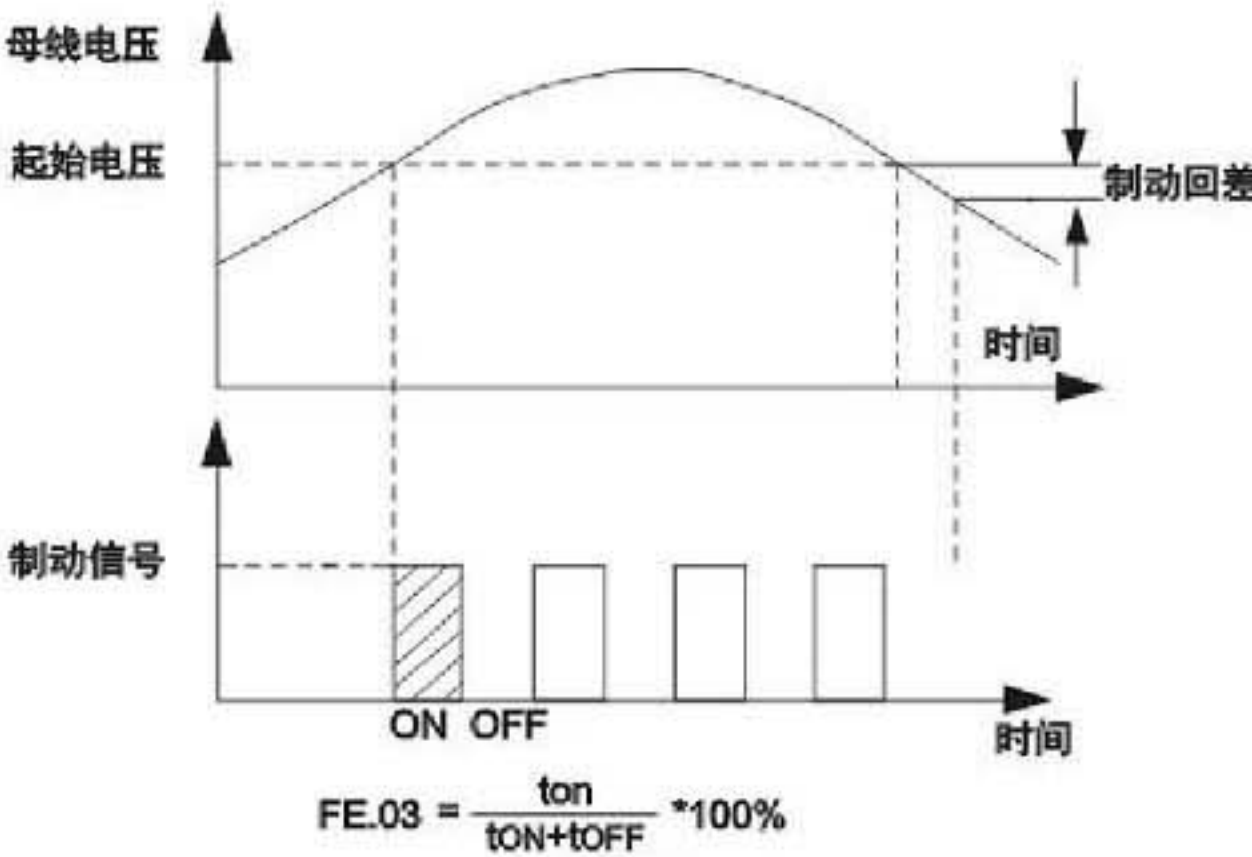
图FE-1 能耗制动示意图
