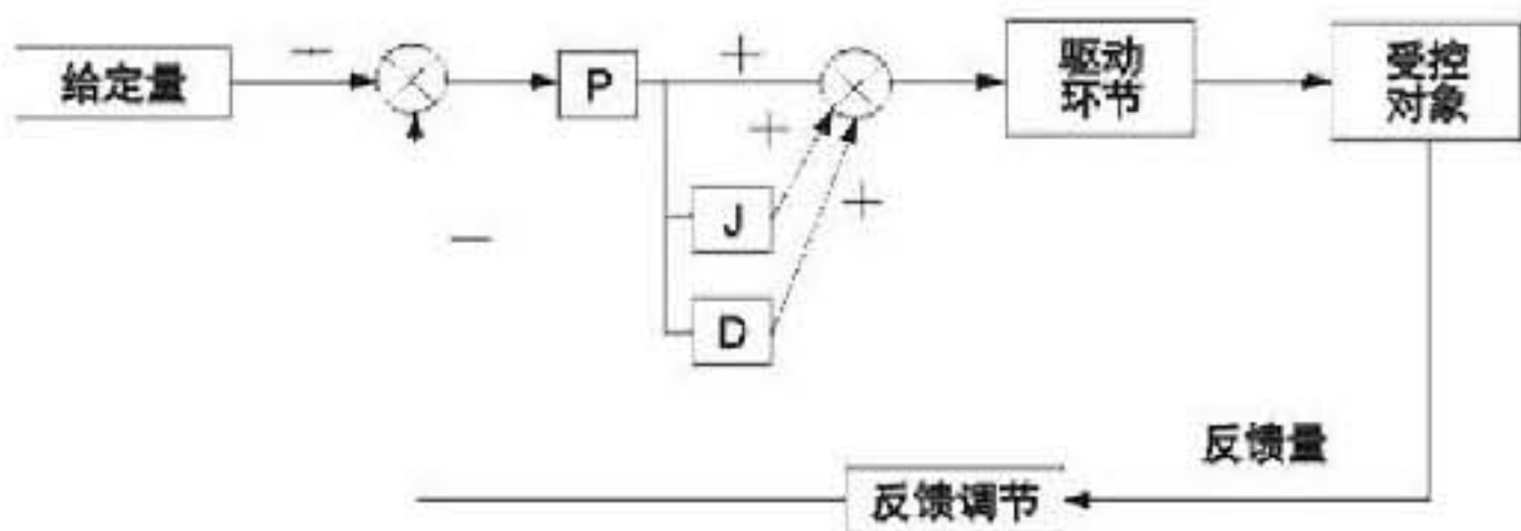
图FA-2 PID调节示意图
