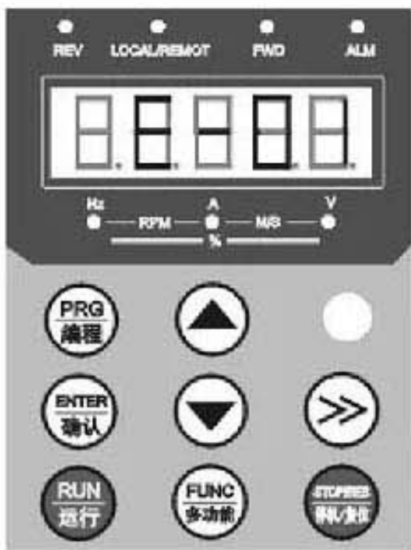
图1-5 加速中过流故障报警显示
