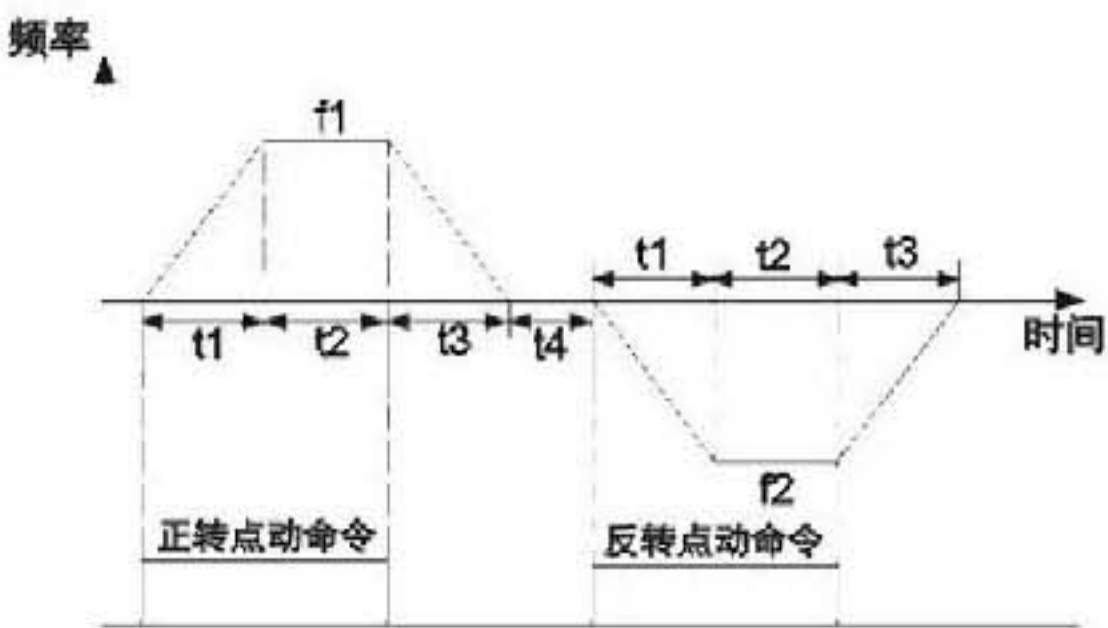
图F8-1 点动运行图
