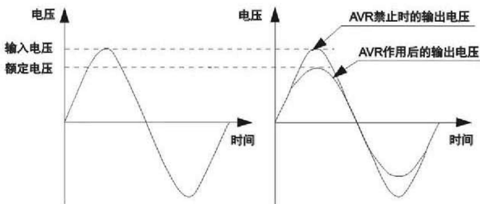
图FE-2 AVR功能示意图
