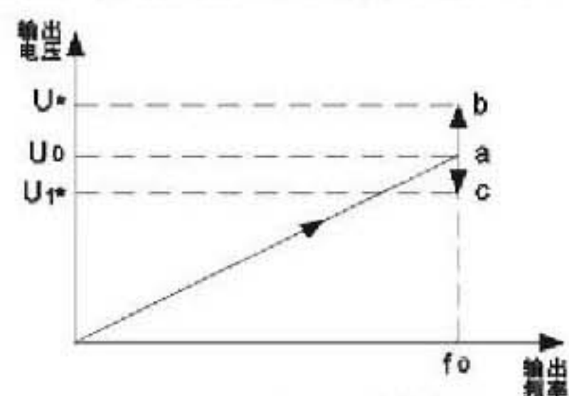
图F3-5 电压控制模式0
