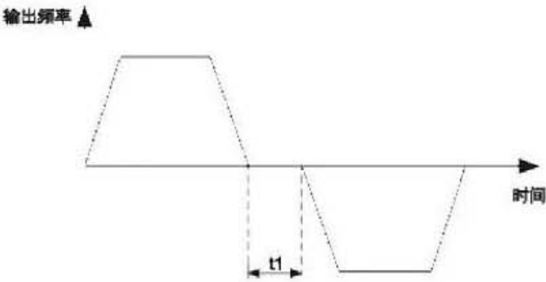
图F8-3 正反转死区时间示意图
