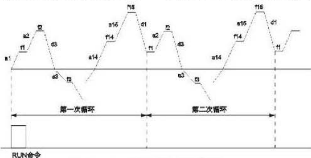
图FC-3 PLC连续循环示意图
