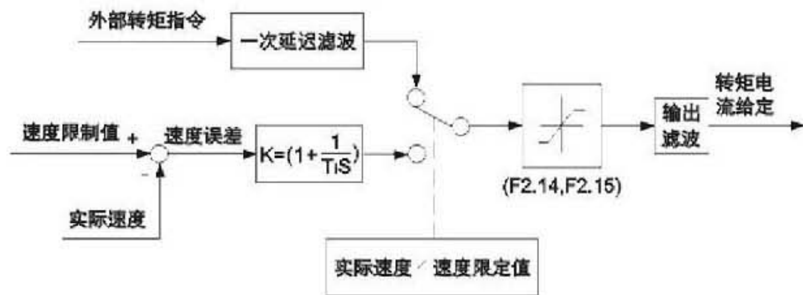
图F2-2 转矩控制简化框图
