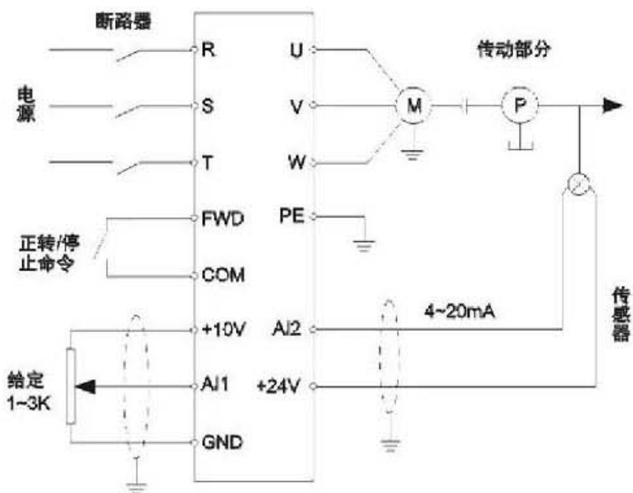
图FA-1 模拟反馈控制系统示意图
