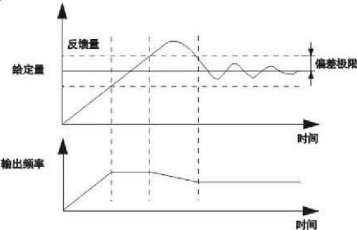
图FA-3 偏差极限示意图
