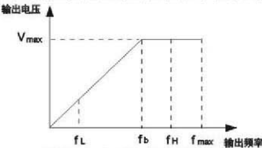
图F0-1 电压与频率示意图
