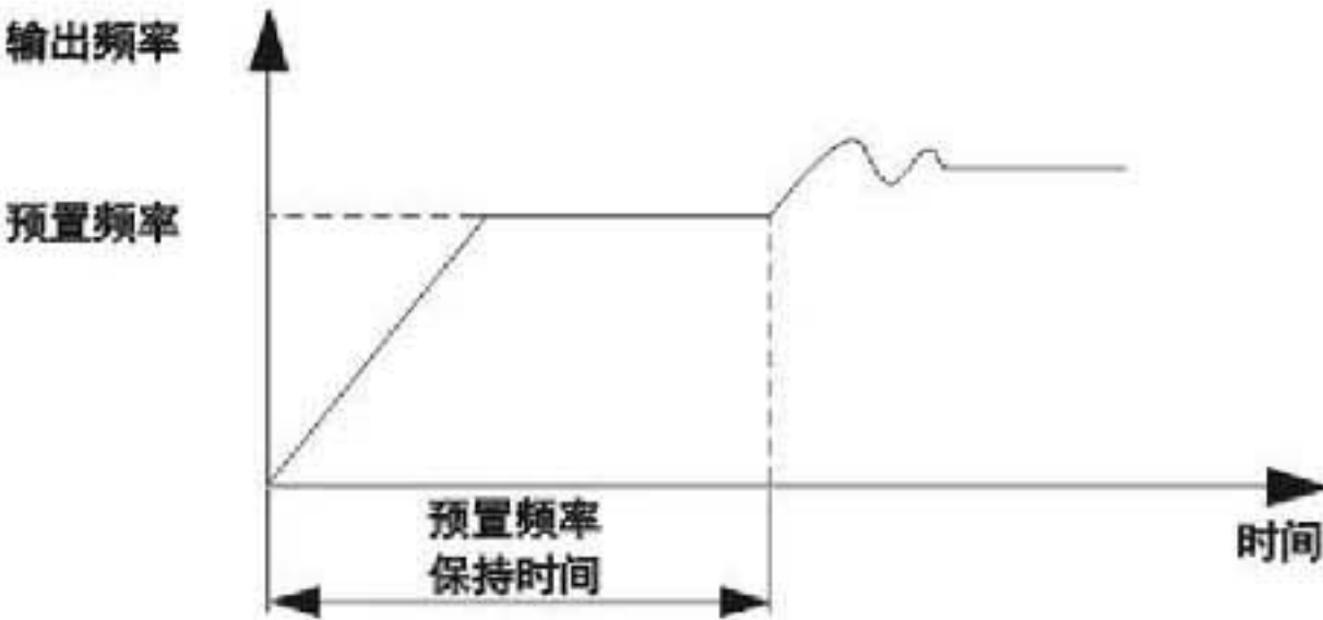
图FA-4 闭环预置频率运行示意图
