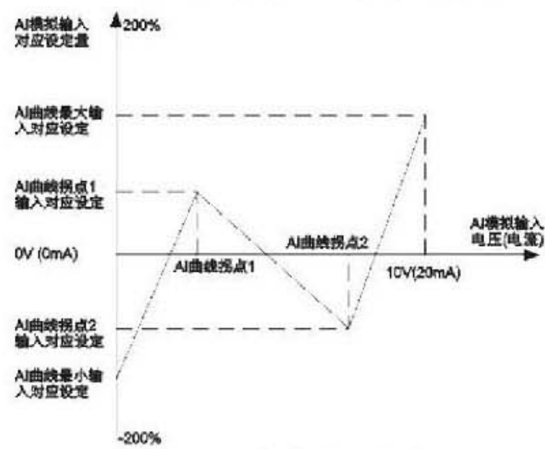
图F4-7 多点曲线示意图
