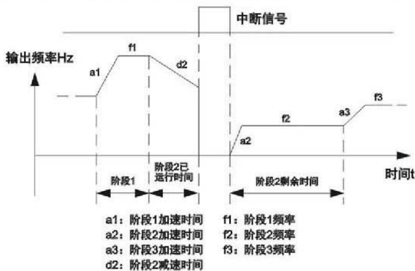
图FC-4 PLC启动方式1
