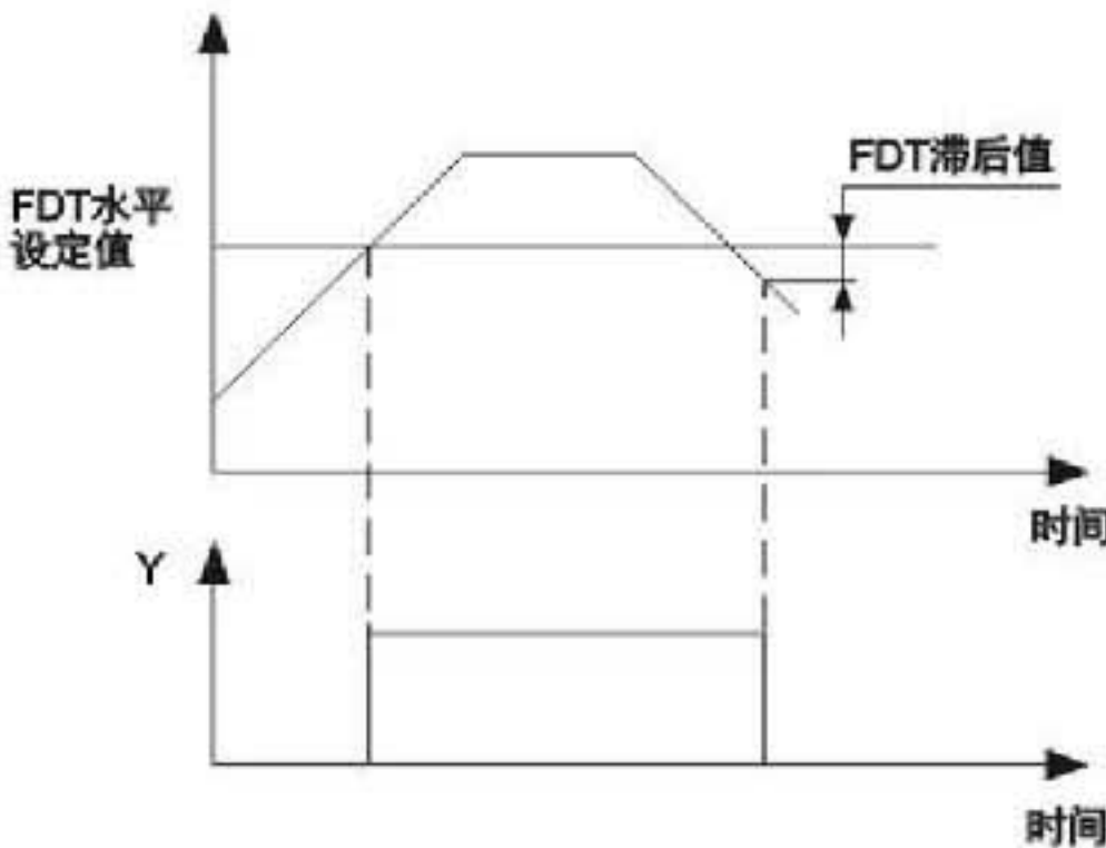
图F8-5 频率水平检测示意图
