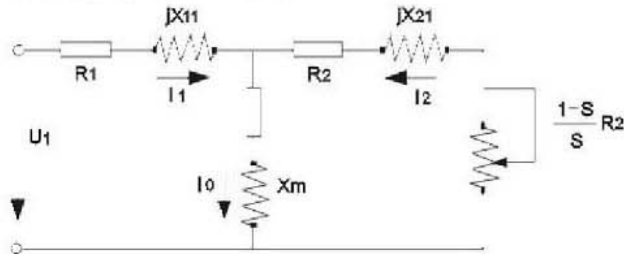
图F1-1 异步电机稳态等效电路图
