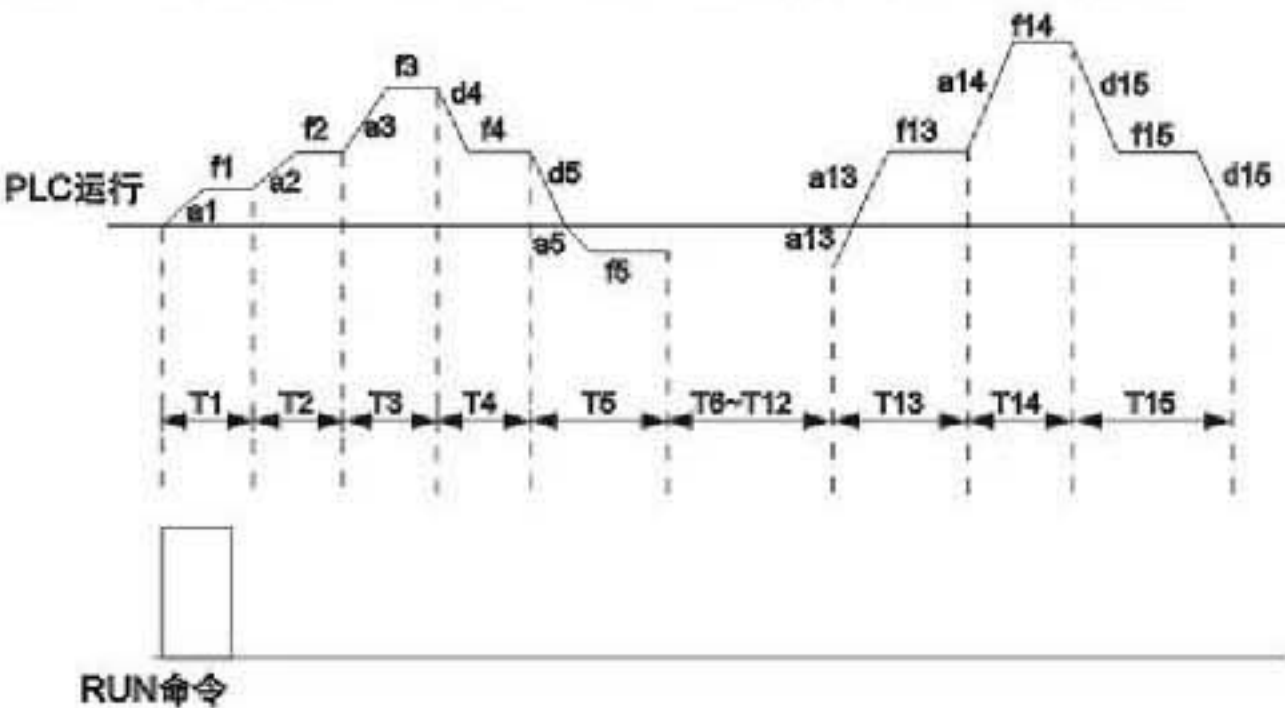
图FC-1 PLC单循环后停机示意图
