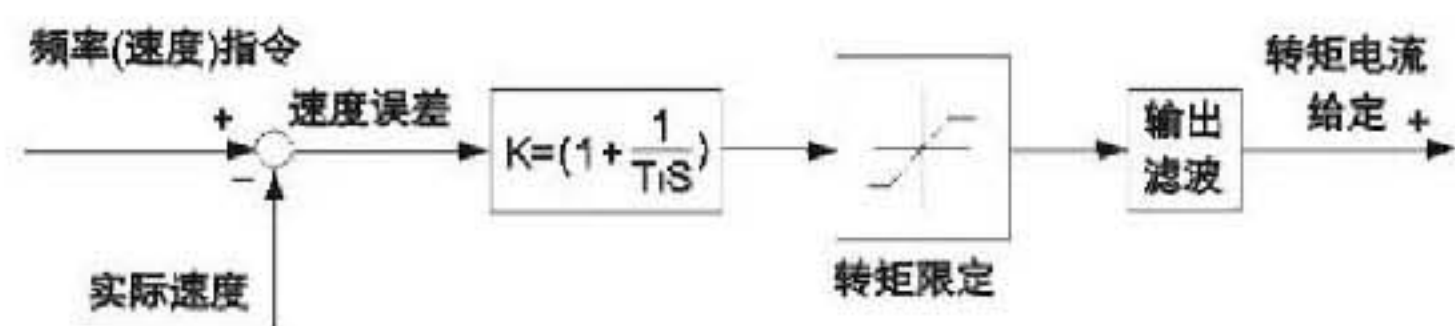
图F2-1 速度调节器简化图
