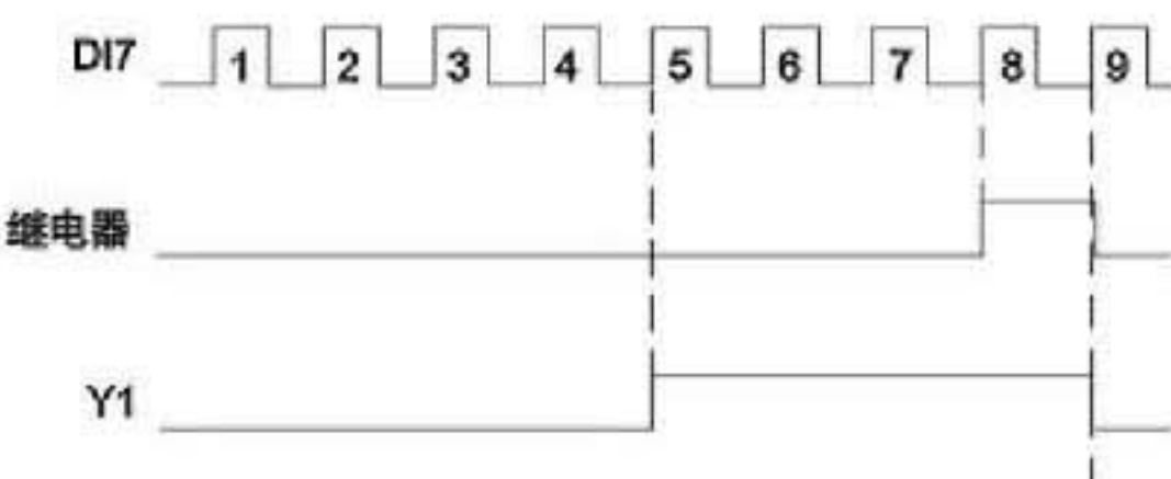
图FB-2 计数器复位设定和计数器检测设定示意图
