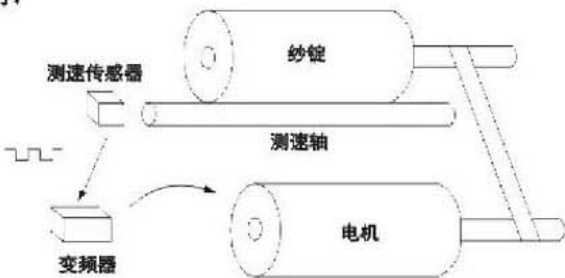
图FB-2 长停机功能举例图
