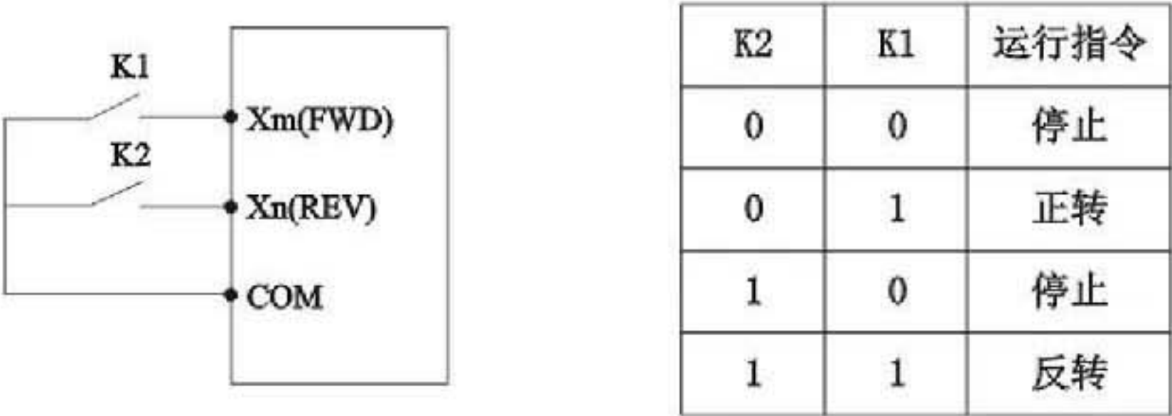
图F4-2 二线式控制模式1示意图
