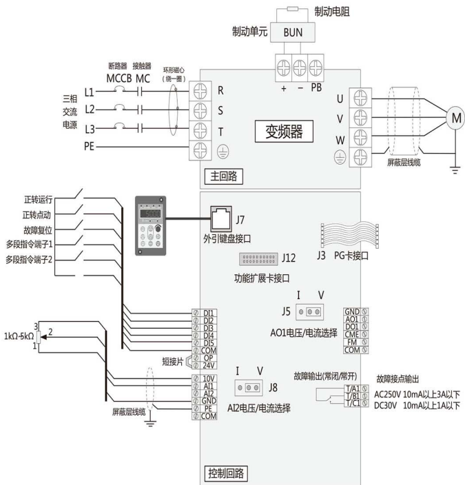
图3-22 变频器电气接线示例
