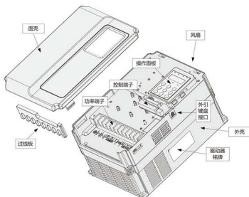
图2-2 变频器塑胶结构外型图
