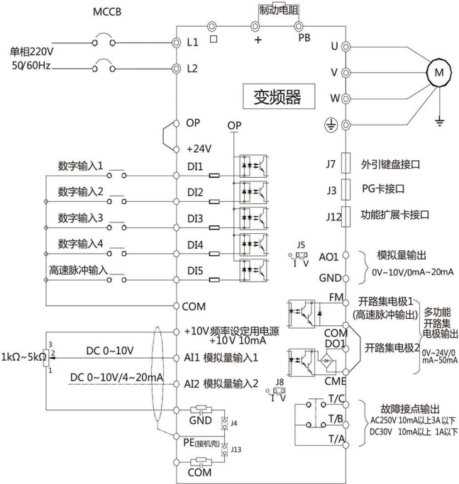
图3-15 变频器控制回路接线方式
