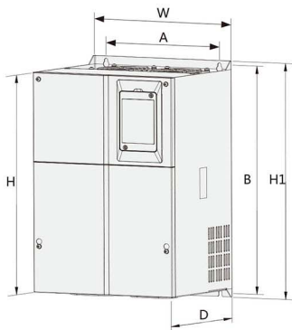
图6-2 钣金结构外型尺寸及安装尺寸示意图
