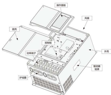
图2-3 变频器钣金结构外型图
