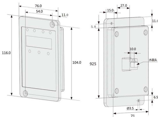
图6-3 外引键盘的外型尺寸（单位：mm）
