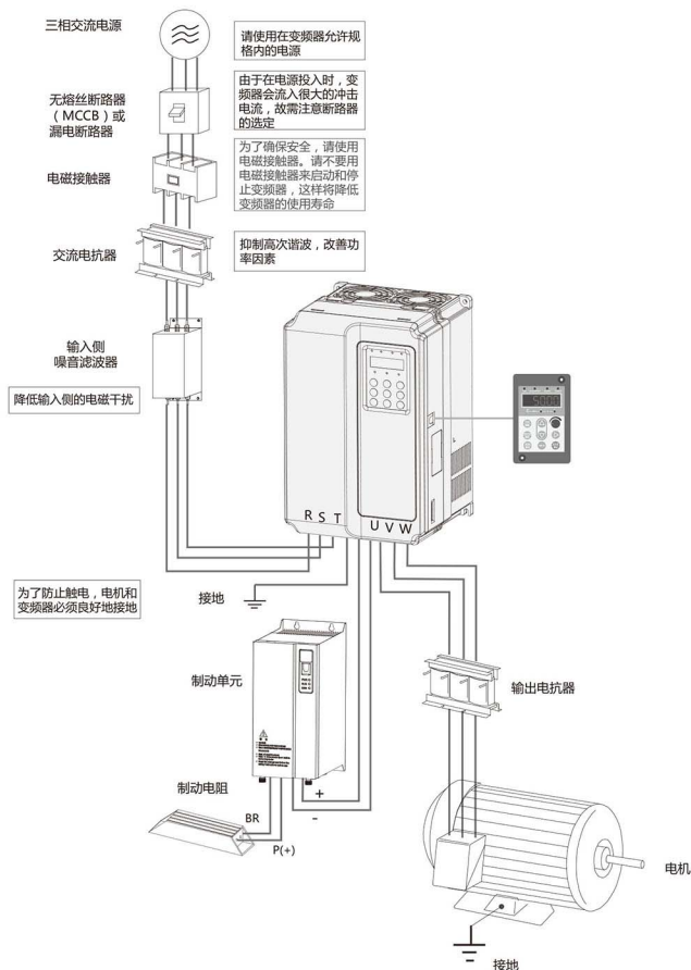
图2-4 系统构成图
