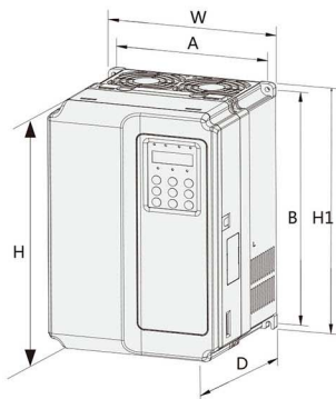
图6-1 塑胶结构外型尺寸及安装尺寸示意图
